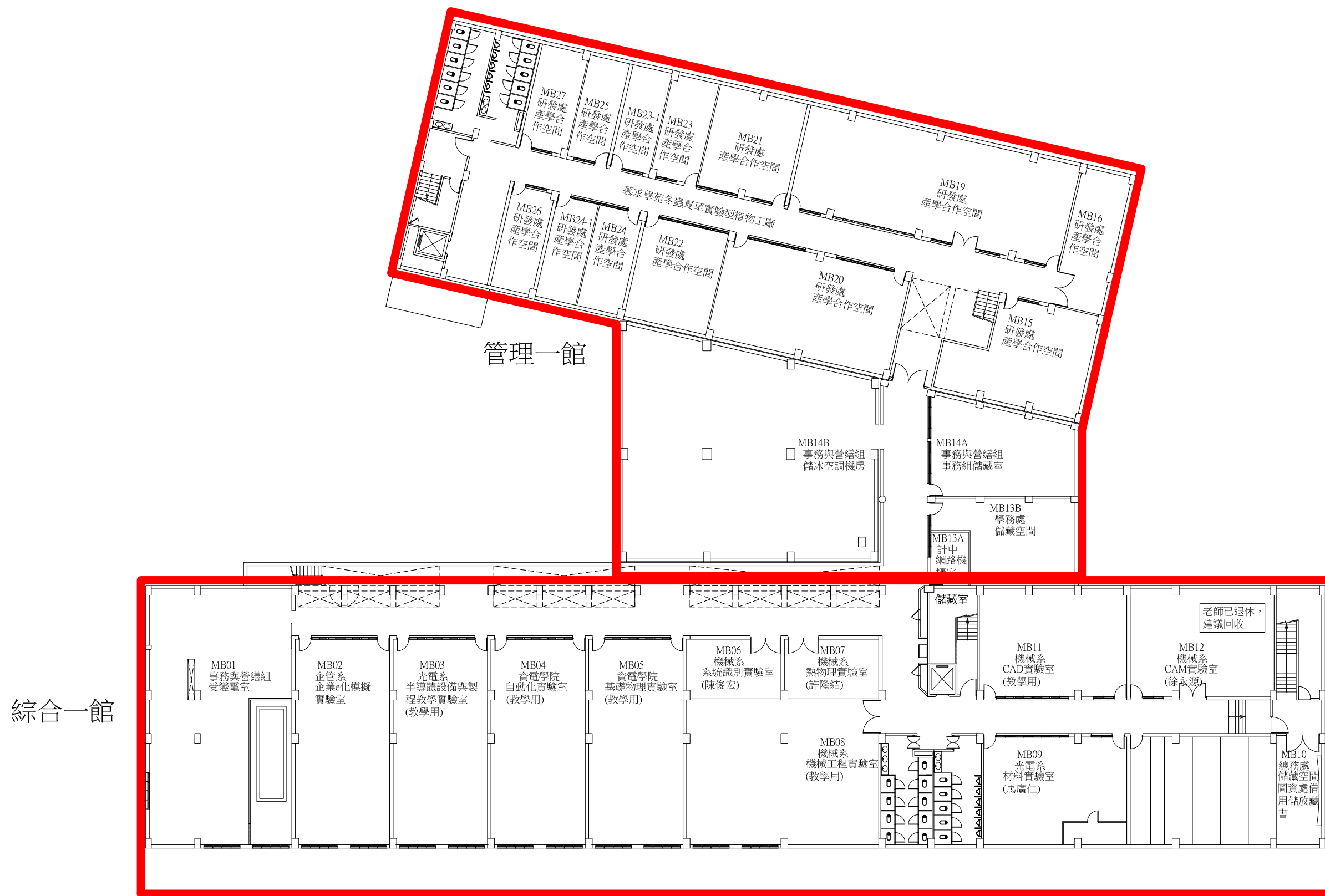
綜合一館暨管理一館地下一層平面圖 S=1/300 (108年01月25日修正版)
